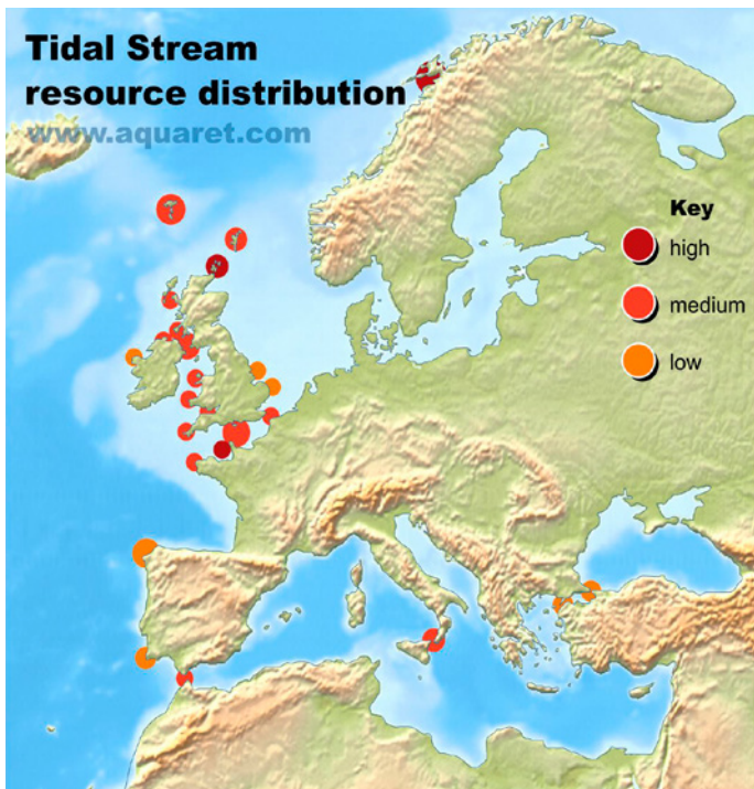
Figura 6.12. Esquema do recurso de fluxo de enerxía da marea en Europa. Imaxe obtida de Aqua-RET (www.aquaret.com)
